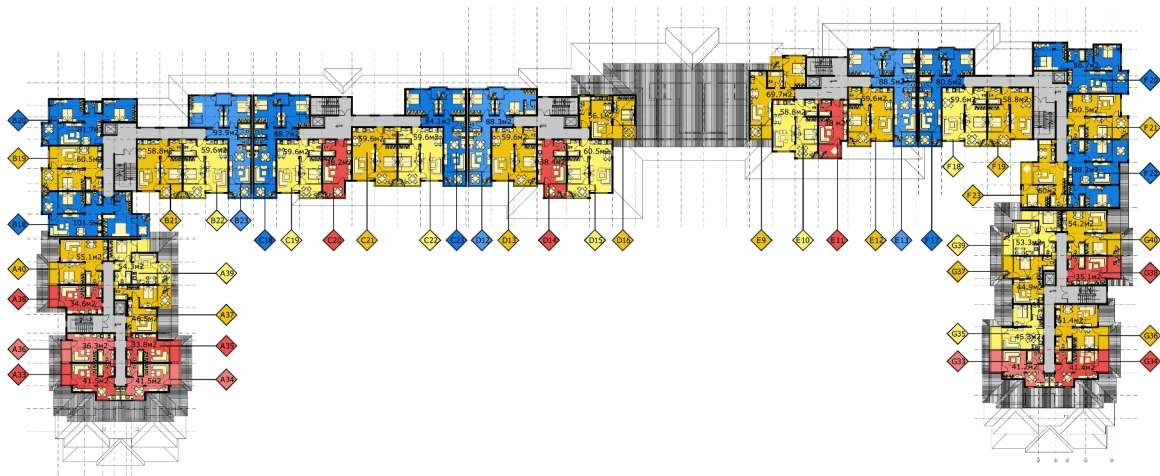
Разпределение на етажа +9.28
