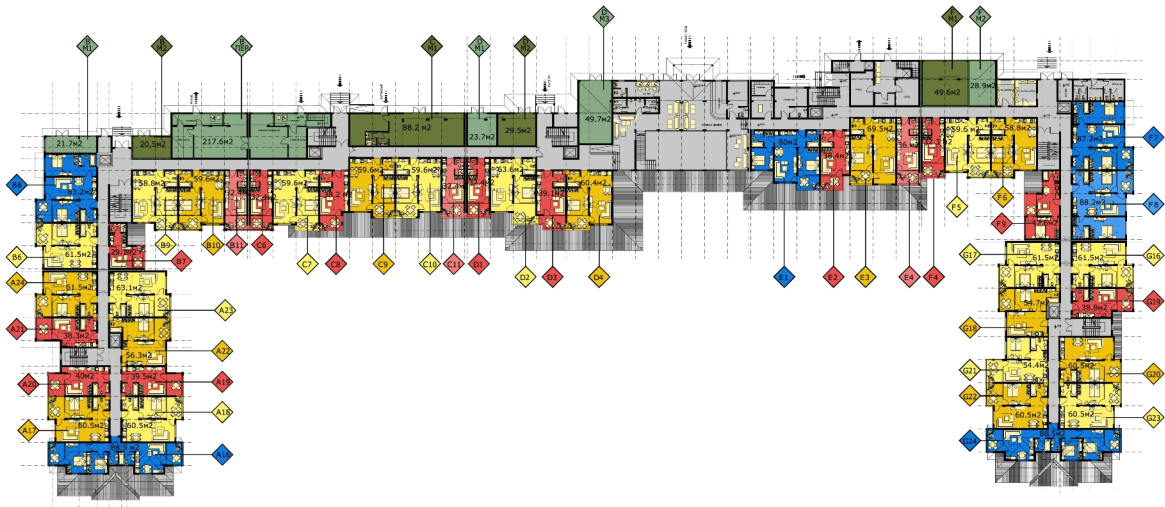
Разпределение на ката \pm 0.00=30.00 и +0.64
