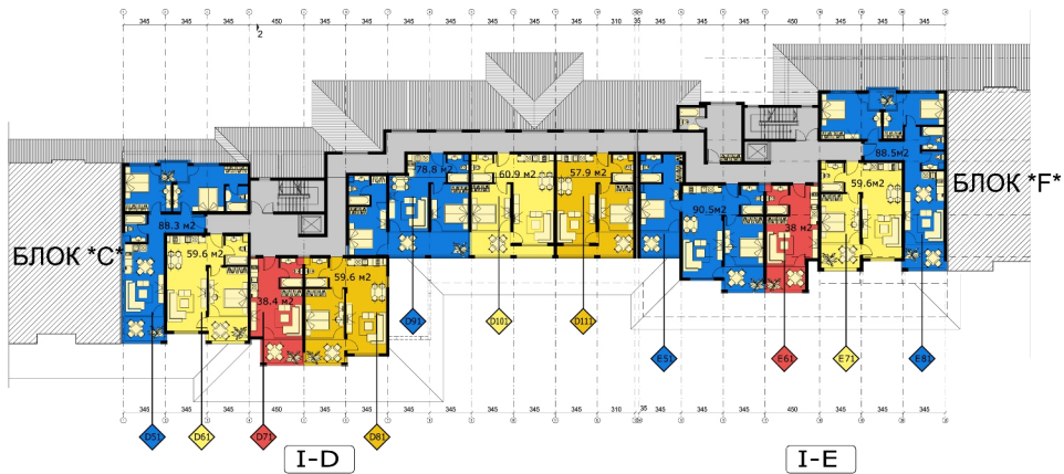
ПЛАН НА КОТА +3.52 FLOOR LEVEL +3.52
