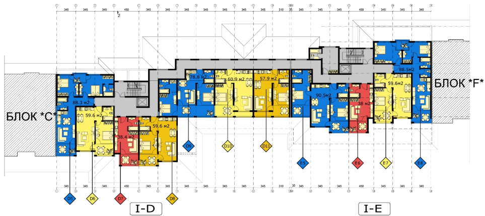
ПЛАН НА КОТА +6.40 FLOOR LEVEL +6.40
